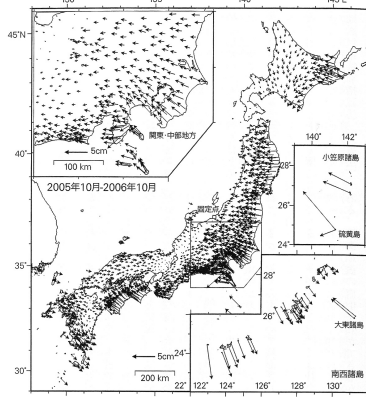
図1-6 GPS観測網により明らかになった日本全国の地殻変動 新潟県大潟観測点(図中に固定点と示す)に対する2005年10月から2006年10月までの各観測点での変動を矢印で示す。
