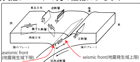
図 0.11 日本の地震とプレートとの関係 [島崎, 1991の図を一部改変] 東北日本では縦ずれ断層が、西南日本では横ずれ断層が卓越
