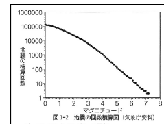
図1-2 地震の回数(震度) (気象庁資料) グーテンベルク-リヒターの関係 (Mが1小さくなると、地震の回数は約10倍になる)
