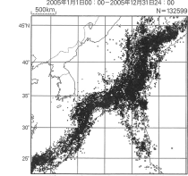
図1-1 2005年1月～2006年10月31日までの日本全国の地震発生回数(マグニチュード1以上、震源10km以内) 1000回以上の地震発生回数を示しているものがある。
