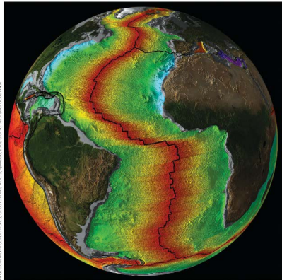
海底の顔い目 大西洋の底にある長さ1万kmに及ぶ「大西洋中央海嶺」は世界最長の山脈だ。色は海底の玄武岩地殻の形成年代を示し、海嶺のそばが最も若く(赤)、大陸に近づくと徐々に古くなっていく。
