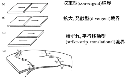
図 1.3 3種のプレート境界。二つのプレートが、(a)がつかり合う、(b)遠ざかる、(c)すれちがう。
