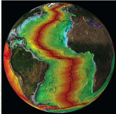
海底の縞い目 大西洋の底にある長さ1万kmに及ぶ「大西洋中央海嶺」は世界最長の山脈だ。色は海底の岩石質地殻の形成年代を示し、海嶺のそばが最も若く(赤)、大陸に近づくにつれ徐々に古くなっていく。
