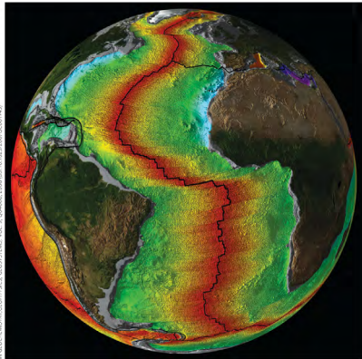
海底の顔い目 大西洋の底にある長さ1万kmに及ぶ「大西洋中央海嶺」は世界最長の山脈だ。色は海底の玄武岩地殻の形成年代を示し、海嶺のそばが最も若く(赤)、大陸に近づくにつれ徐々に古くなっていく。
