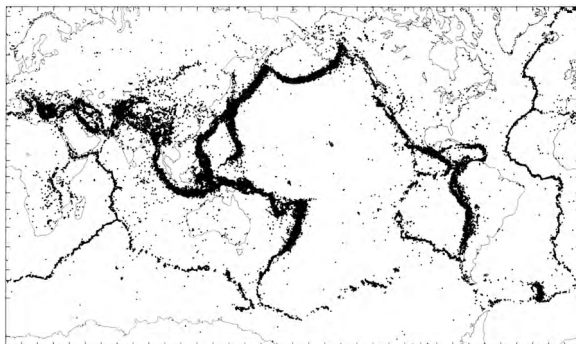
図 4.28 世界の地殻分布図 (M28-4.0、深さ 100 km 以下、1980-1998 年、国際地震センター作成)
