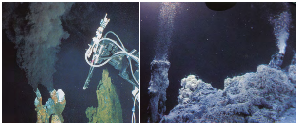
Black smoker (東太平洋海嶺)
